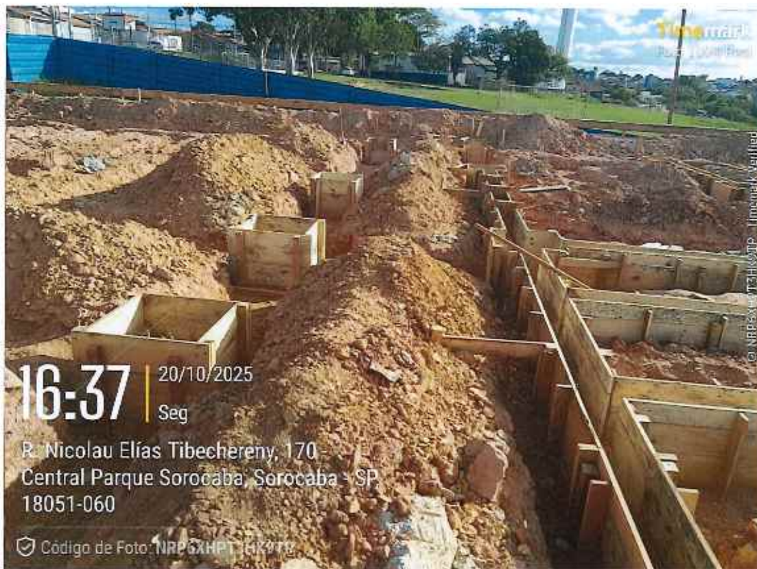
Execução de forma de vigas balcrame
